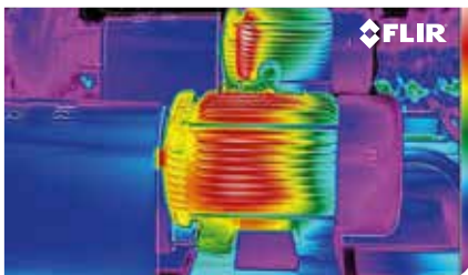
Kontinuierliche Überwachung eines Motors.
